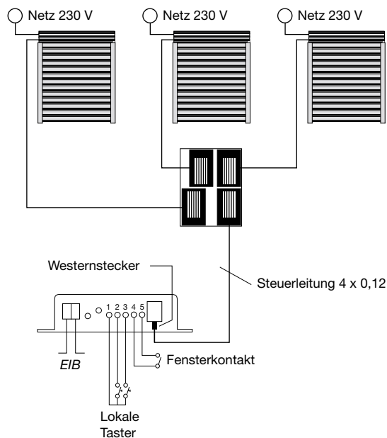
Parallelschaltung von bis zu 3 Antrieben mit Hilfe des Adapters Westernstecker/Westernstecker
