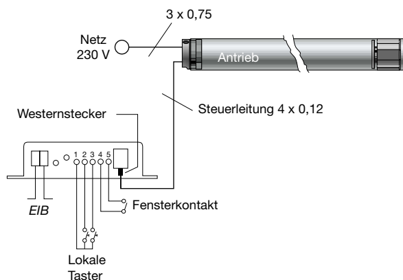
Anschlußbild Antrieb und Interface
